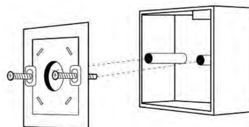
Modo empotrar
