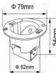
base independiente
