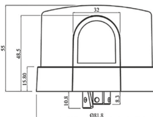
SENSOR PARA FAROLA 4400030
